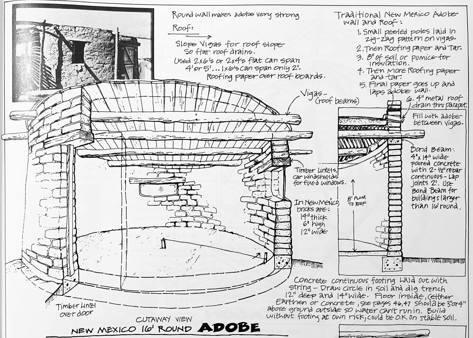
Fig. 5 - Illustrazione di un'abitazione circolare in mattoni di argilla. Tratto da Shelter, copyright 1973 by Shelter Publications, Inc. Ristampato con permesso. Shelter Publications/AdventureKEEN.
