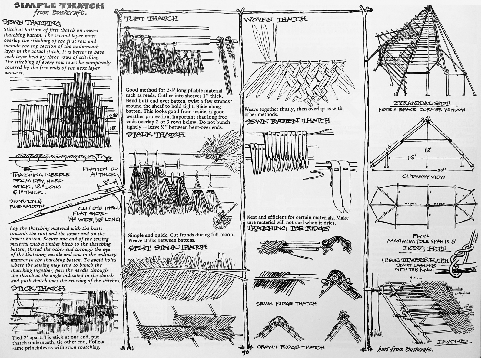
Fig. 3 – Tecniche per realizzare tetti intrecciati. Tratto da Shelter, copyright 1973 by Shelter Publications, Inc. Ristampato con permesso. Shelter Publications/AdventureKEEN.
