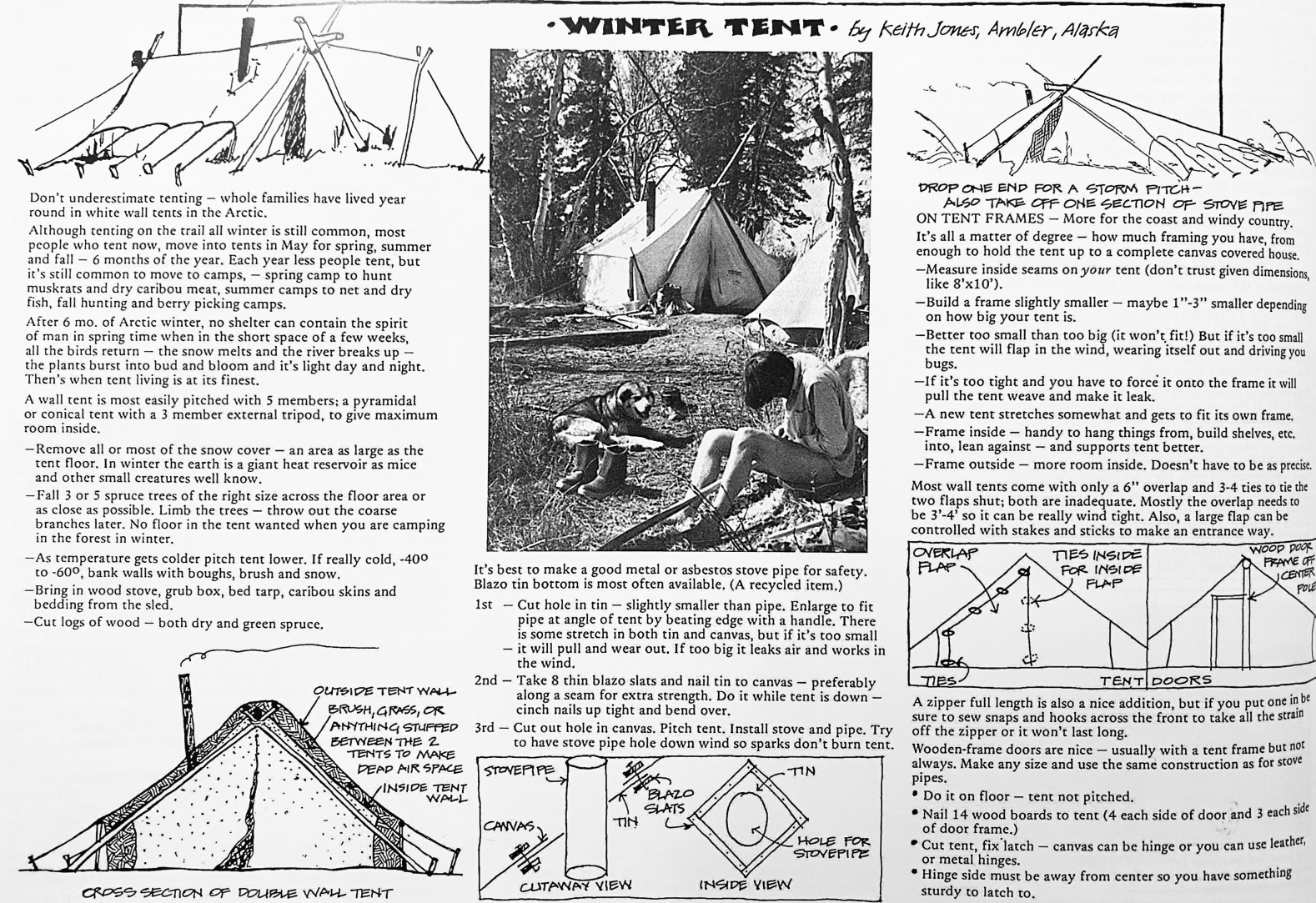
Fig. 2 – Possibili tipologie di tende invernali. Tratto da Shelter, copyright 1973 by Shelter Publications, Inc. Ristampato con permesso. Shelter Publications/AdventureKEEN.
