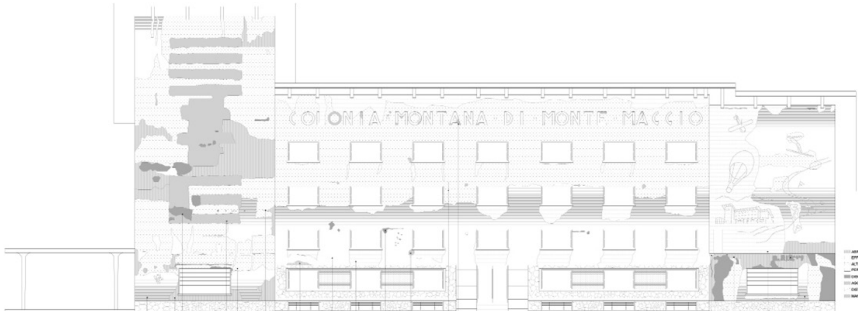
fig. 45 La Colonia di Monte Maggio: il degrado materico dei fronti, scala originale 1:50.
